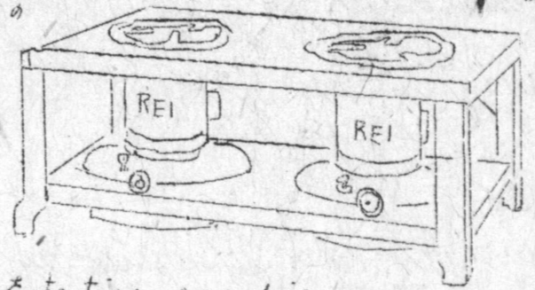
Este tipo, com dois queimadores e de pés baixos, é geralmente usado por pequenas famílias de 2 a 3 pessoas. Pesa 6 1/2 Kgs. e sua mesa mede 60 x 30 cm. com 24 cm. de altura
